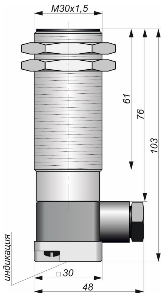
Габаритный чертеж
